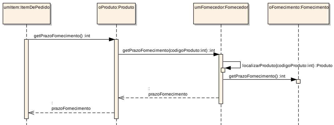
Figura A.24: Uma solução de colaboração para obtenção do prazo de entrega de um pedido feito à ZYX.
