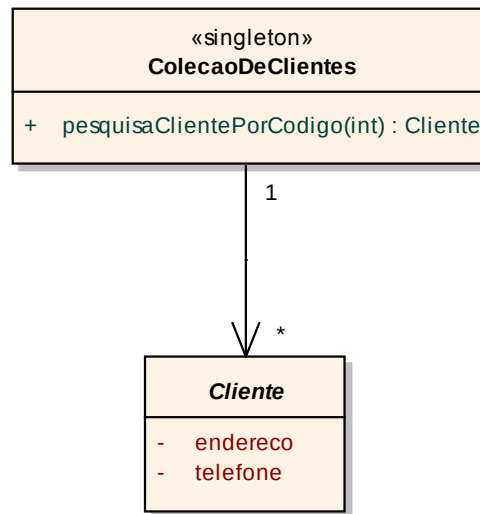
Figura 9.3: Incorporação de classe de projeto ao diagrama conceitual.
